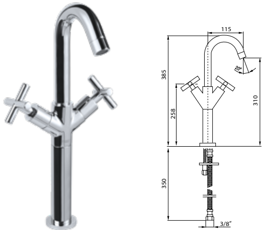
40 102 ●●●● Monobloc lavabo alto Single-hole high wash-basin Mélangeur lavabo haut monotrou 1-loch-zweigriff-waschtischbatterie hoher Высокий смеситель для раковины
