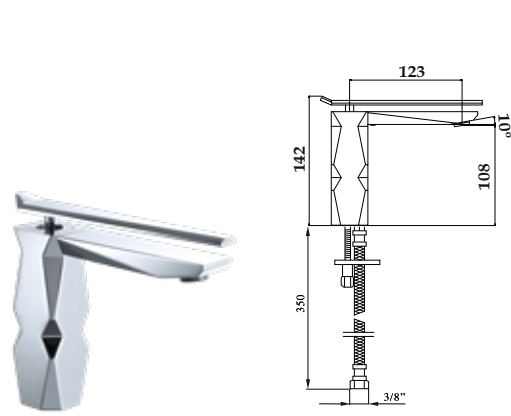
74 002 ●●●●●●●● Monomando lavabo Wash-basin mixer Mitigeur lavabo Einhebel waschtischmischer Однорычажный Смеситель для раковины
