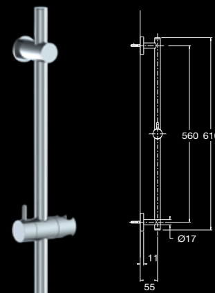
21 118 ●●●●●●●●●● Barra deslizante de ducha redonda latón Shower sliding bar round brass Barre de douche glissant laiton ronde Brausestange runden messing Душевая штанга круглая из латуни
