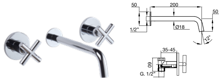
40 305 ●●●● Bimando lavabo empotrado Concealed 3 holes wash basin mixer Mélangeur de lavabo 3 trous à encastrer Unterputz 3-Loch Waschtischmischer Встроенный смеситель для раковины на 3 отверстия
